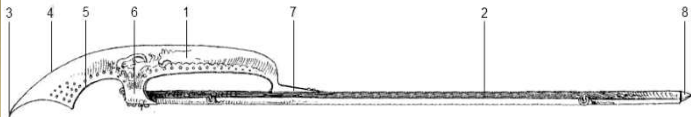
Конструкция бердыша
